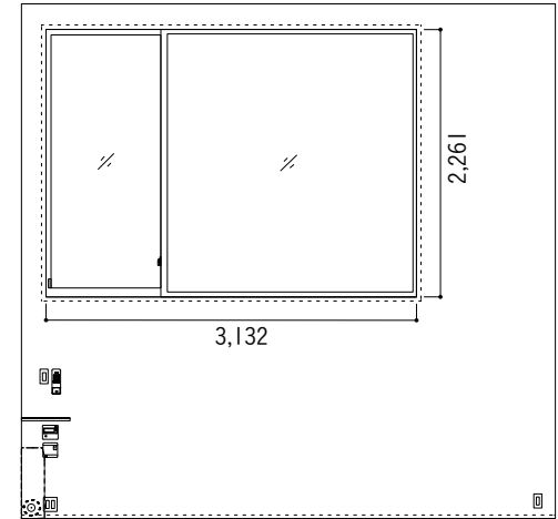
西側壁面
